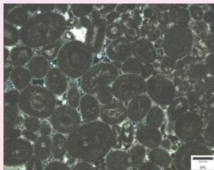
Dunham: Grainstone
